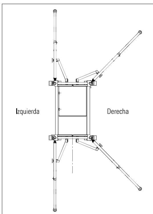
Montaje lateral
